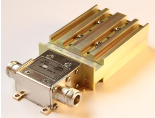
L-Band 1.5 Kw CW isolator
